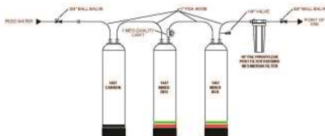
MIXED BED DI SYSTEM
